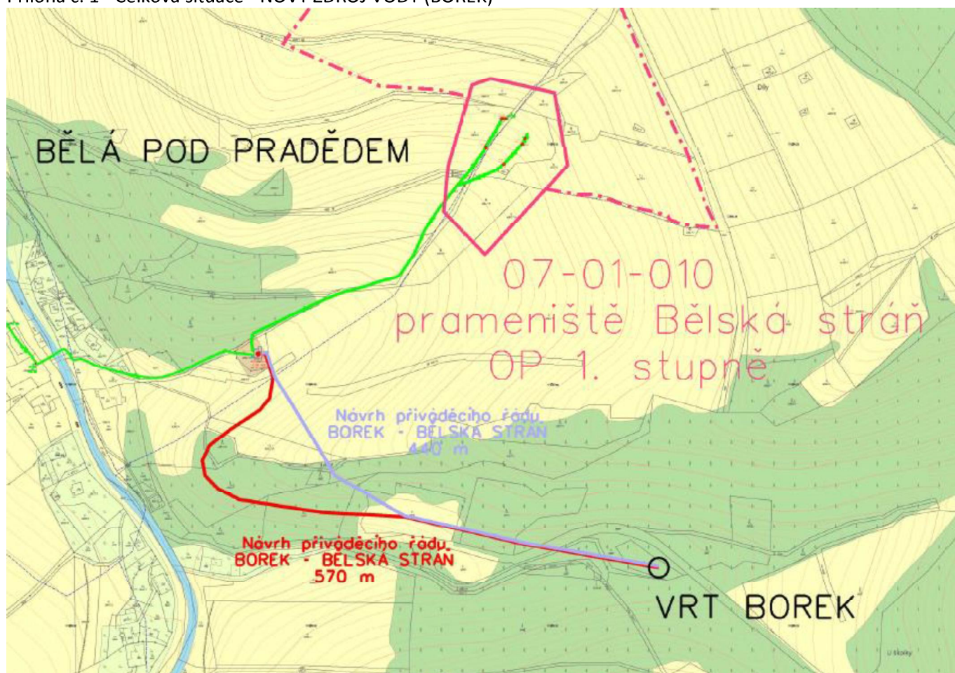
Příloha č. 1 - Celková situace - NOVÝ ZDROJ VODY (BOREK)
