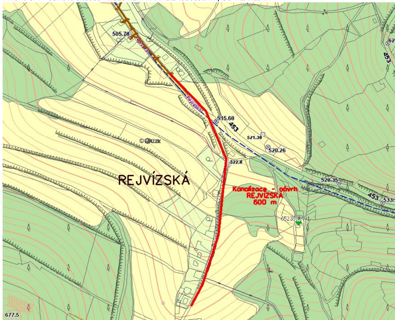
Příloha č. 4 - Celková situace - ROZŠÍŘENÍ KANALIZACE JESENÍK, UL. REJVÍZSKÁ
