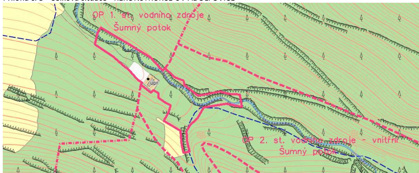
Příloha č. 5 - Celková situace - REKONSTRUKCE ÚV ADOLFOVICE
